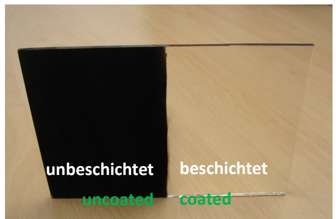
Beschichtete Seite: Rußabbau ab 300 °C Coated side: Soot removal from 300 °C
